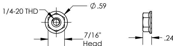
3) Nut, Flange Hex 1/4-20
